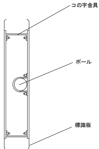
取付け断面図
