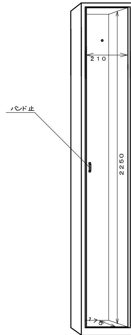
内 寸
