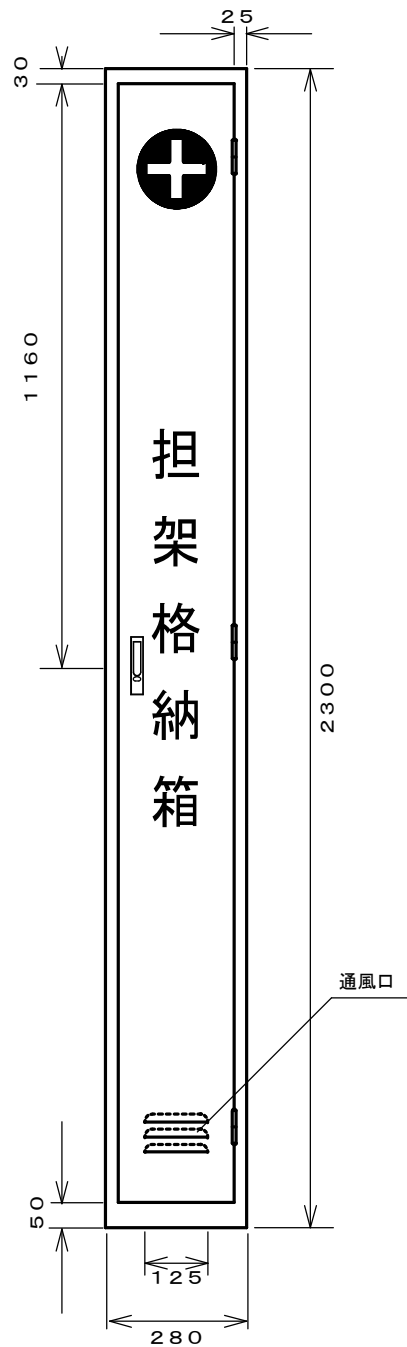
正面図
